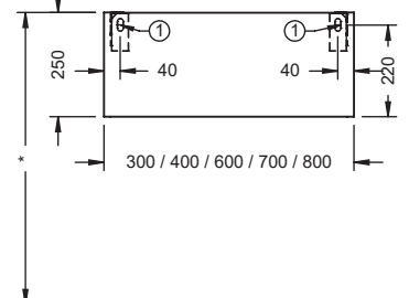
* Maß abhängig von Abdeckplatte und Waschtisch
