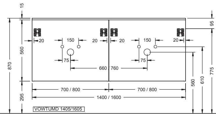
Linke Version abgebildet, rechte Version spiegelbildlich.
