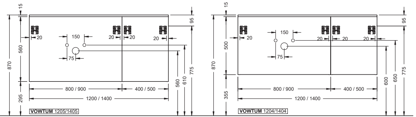
Linke Version abgebildet, rechte Version spiegelbildlich.
