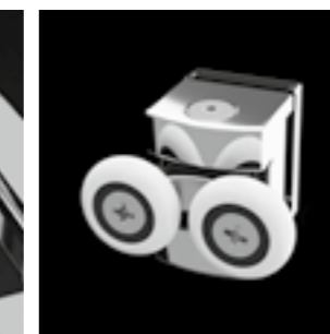
Verstellbare Rollen zur passgenauen Einstellung der Türen
